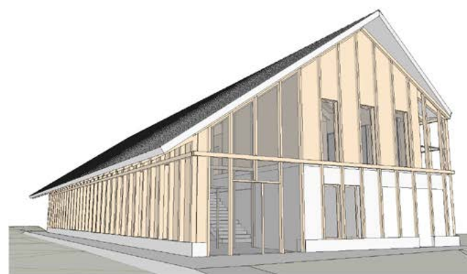
Les différentes façades de la Maison de santé pluridisciplinaire
